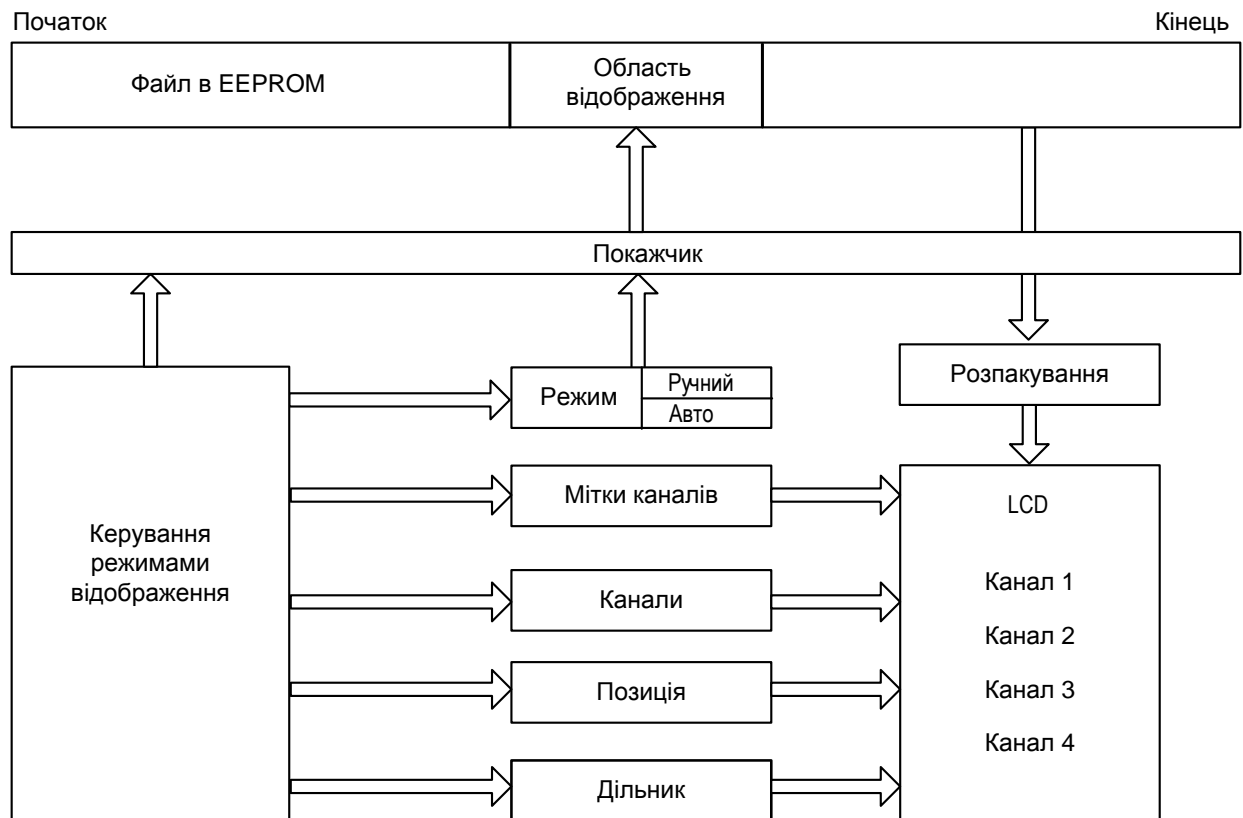
Рисунок Х.Х - Функціональна схема осцилографа
